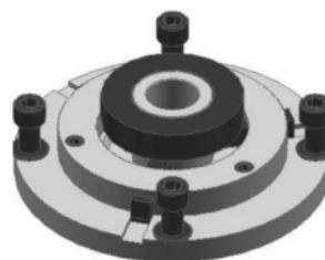
AC1177 Univerzální adaptér pro brzdový buben D1: 220÷250 mm, D2: 275 mm, N: 8
