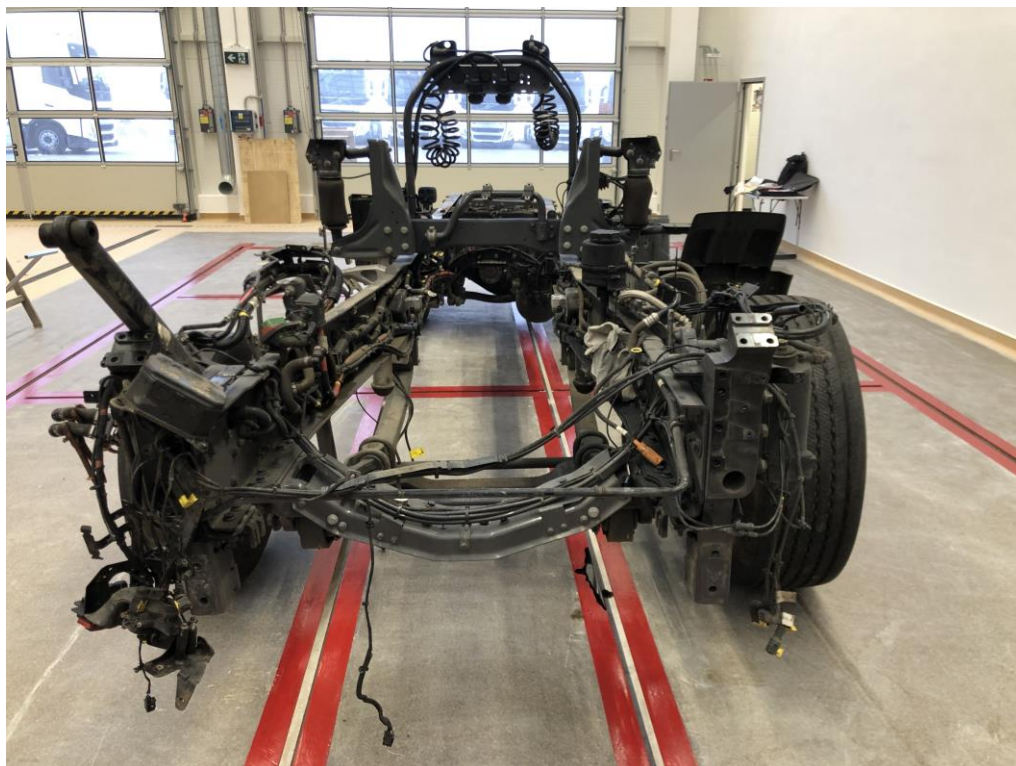
Josam - pracoviště pro měření a rovnání rámců a kabin
