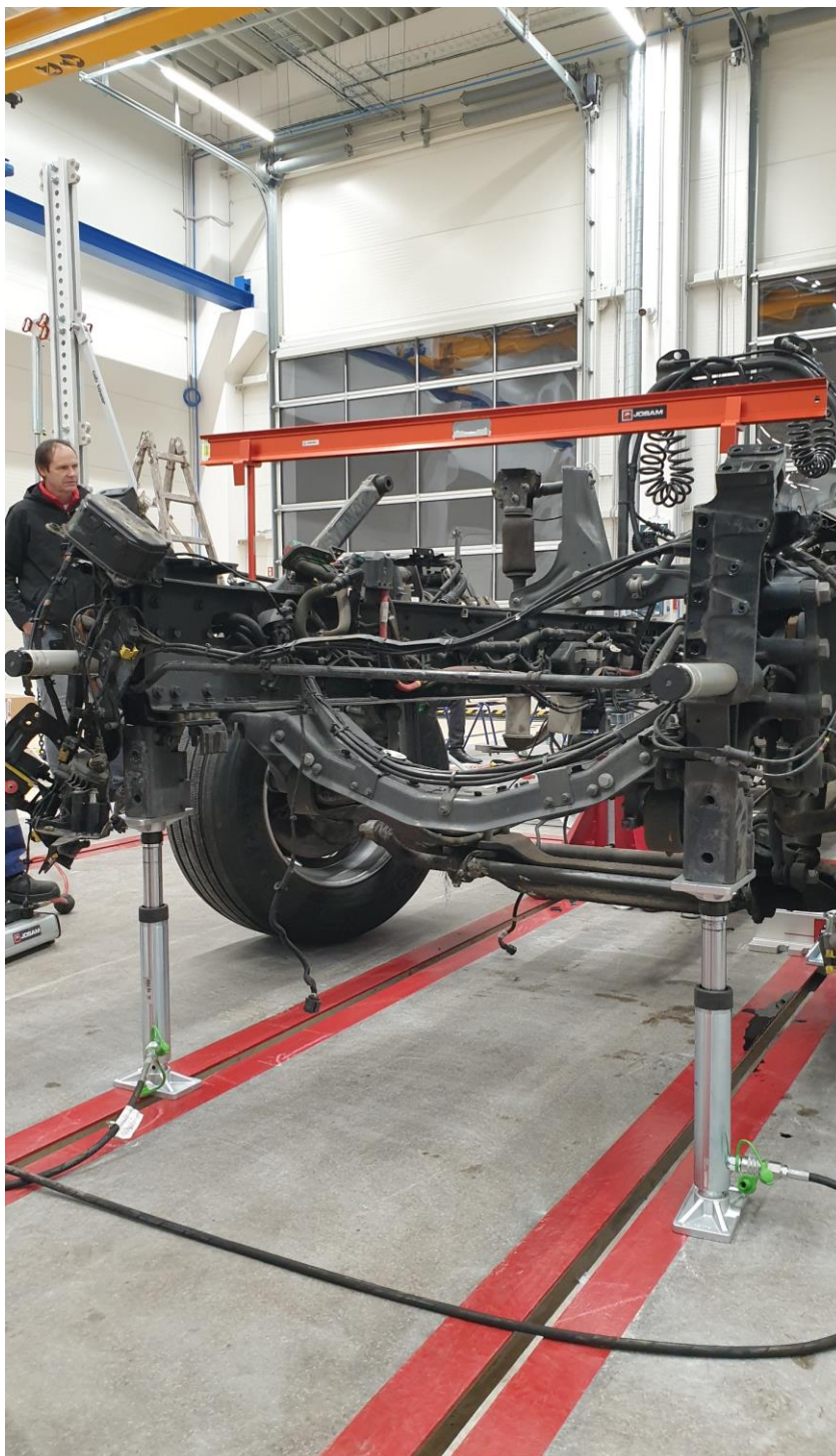
Josam - rovnání a měření rámu
