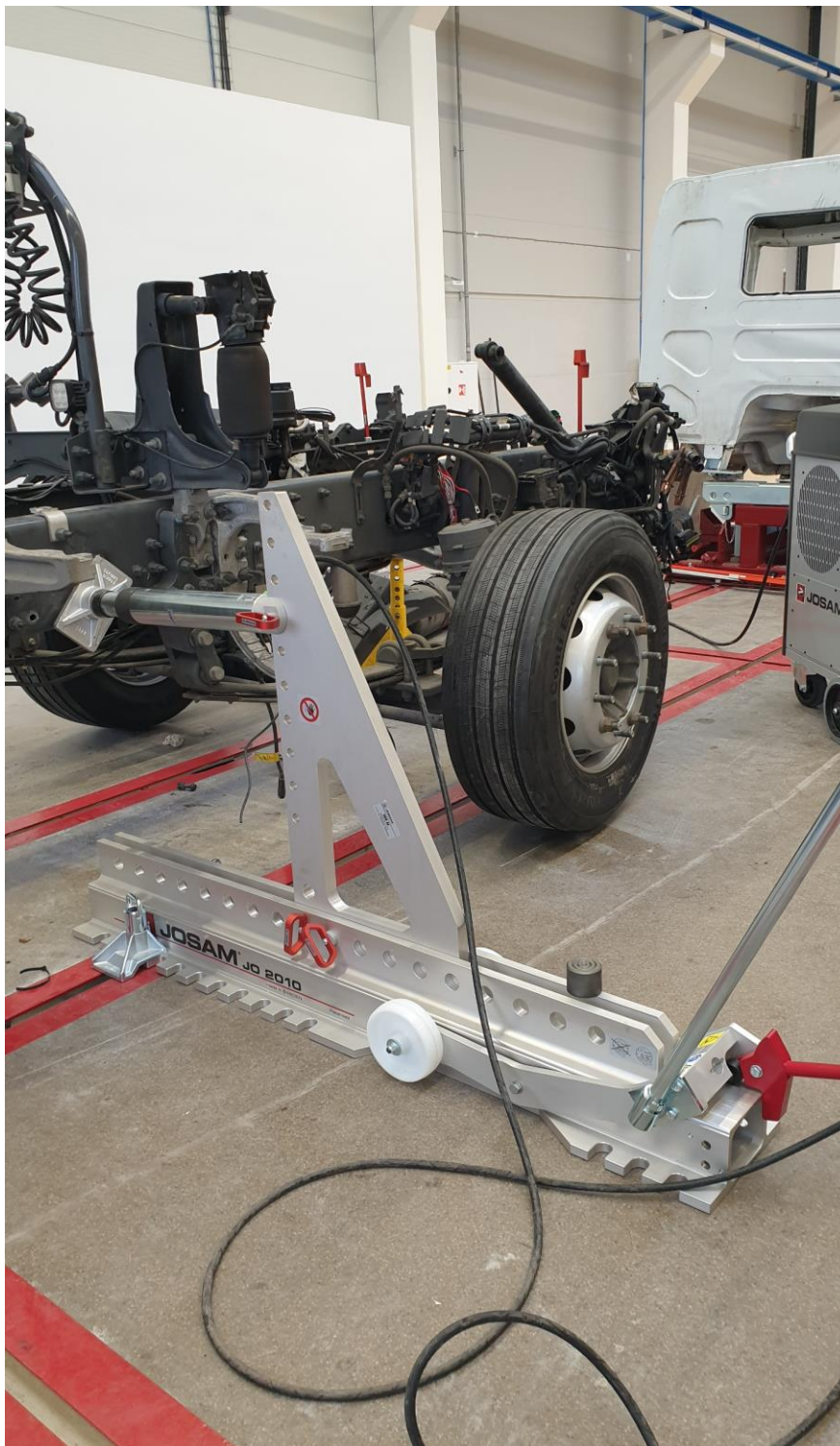
Josam - rovnání a měření rámu
