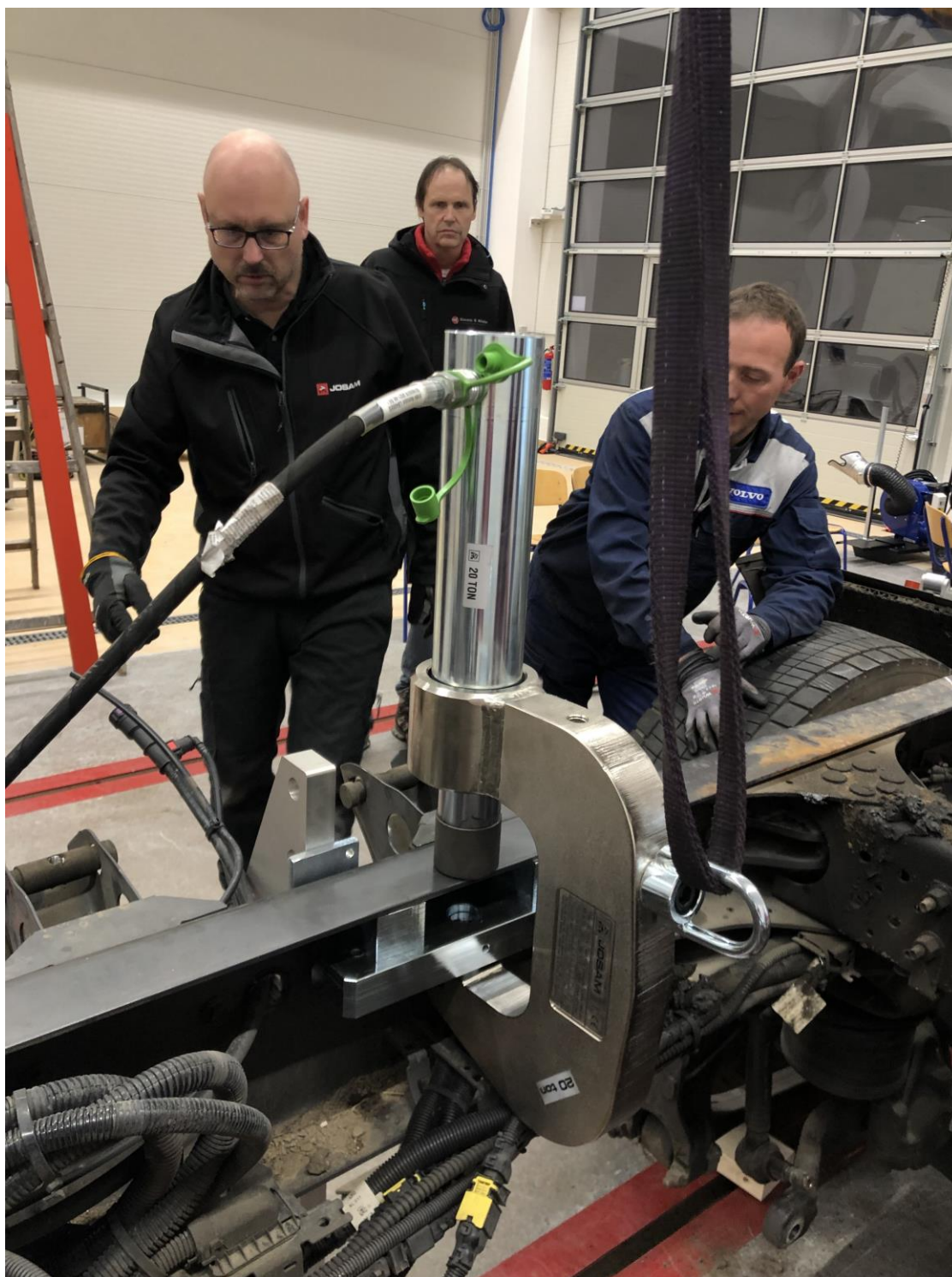
Josam - oprava poškozeného rámu pomocí hydraulické „C“ klemy
