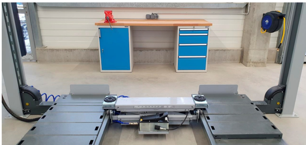
SPACE SQ 502 L - 4 sl. zvedák 5 t pro měření geometrie dodávek + Z37 - přízved nápravy 2 t
