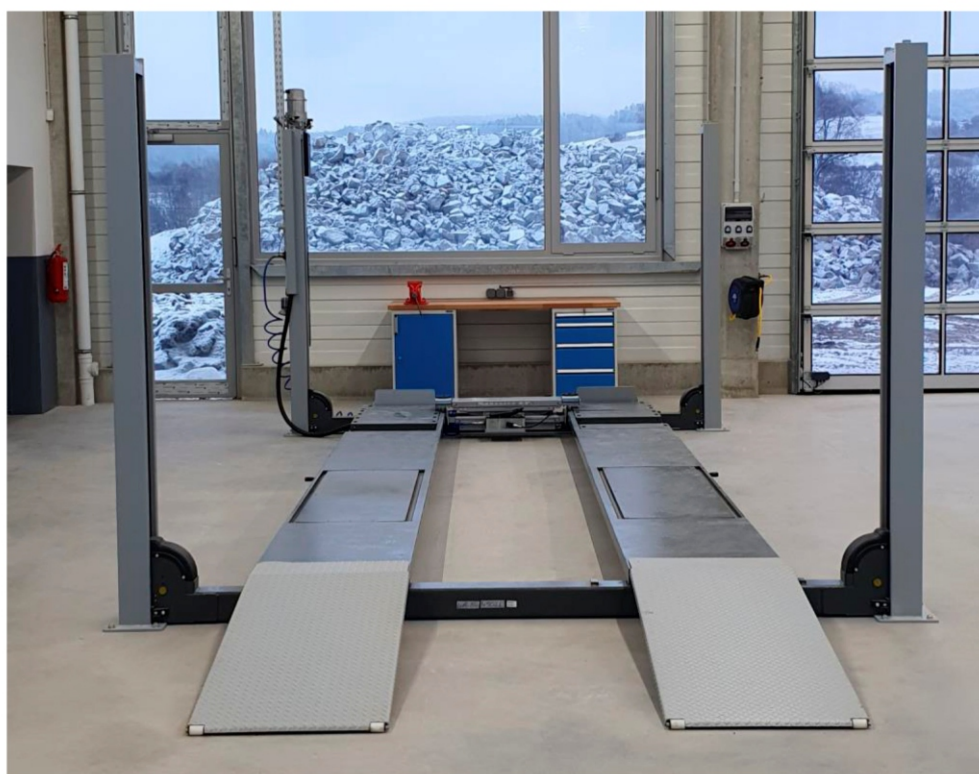
SPACE SQ 502 L - 4 sl. zvedák 5 t pro měření geometrie dodávek + Z37 - přízved nápravy 2 t
